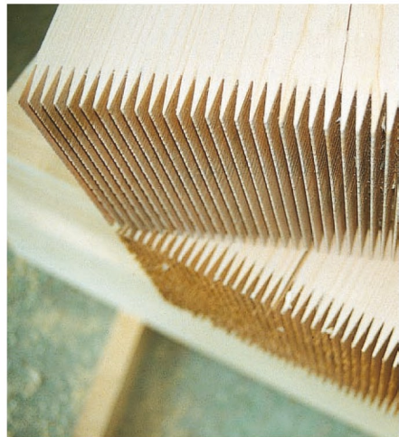
Keilzinkenverbindung
